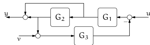
(א) דיאגרמת בלוקים
