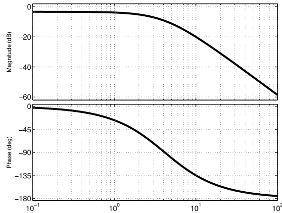
איור 13: דיאגרמת בודה לשאלות מס' 65 ו-66
