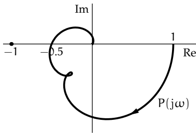
(ג) תיאור פולרי לשאלה מס' 55
