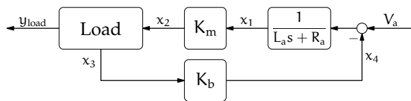
(ב) מנוע זרם ישר
