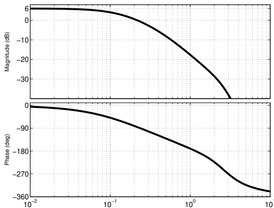
(ב) דיאגרמת בודה לשאלה מס' 57
