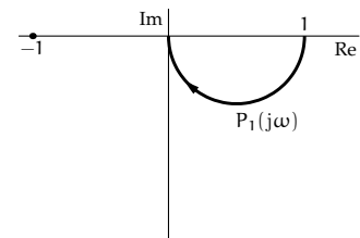
(א) P_1(s)
