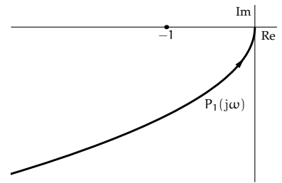
P_1(s) (א)
