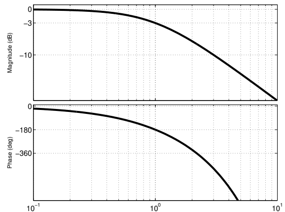
(א) דיאגרמת בודה לשאלה מס' 56
