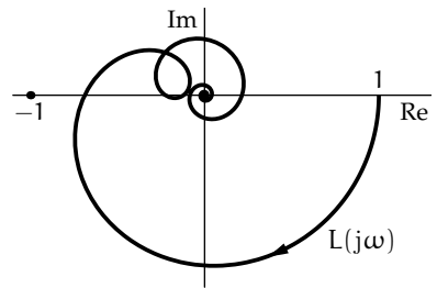
(א) תיאור פולרי לשאלה מס' 53
