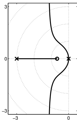
(ג) מג"ש לשאלה מס' 47
