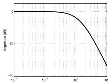
(ה) G_2(s)
