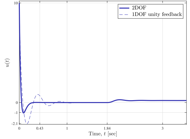
(d) Control input signal
