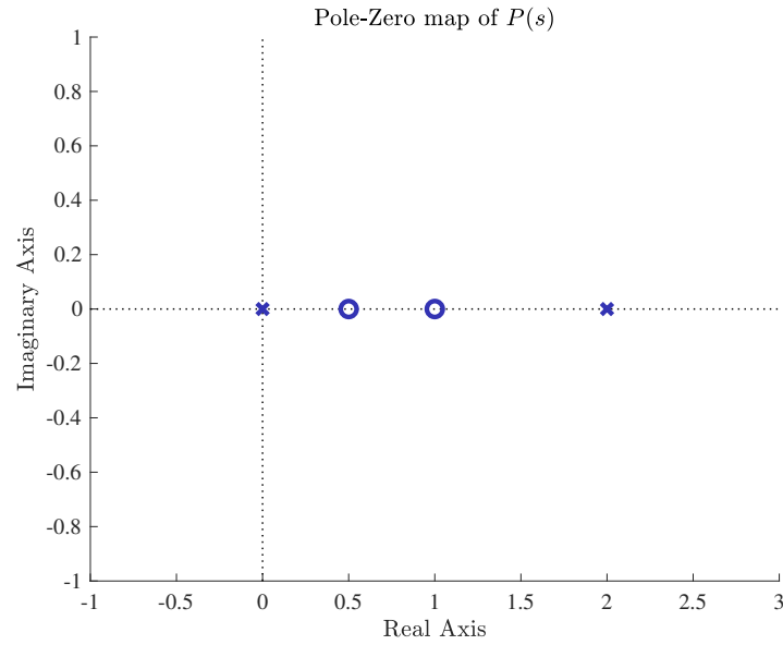
איור 13: מפת הקטבים של התהליך
