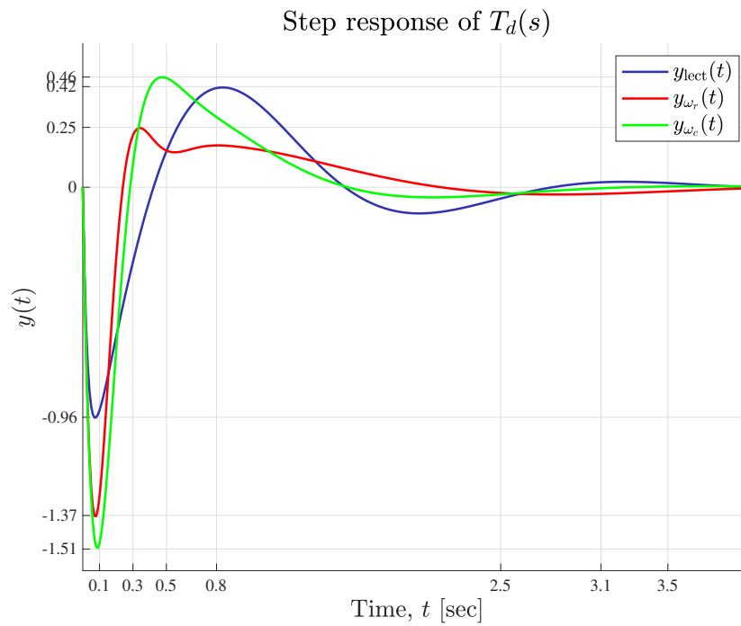
איור 6: תגובת שלושת החוגים להפרעת מדרגה
