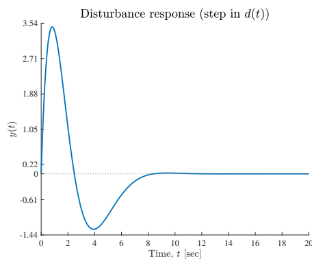
(א) תגובת ההפרעה עבור צמצום של אפס איטי
