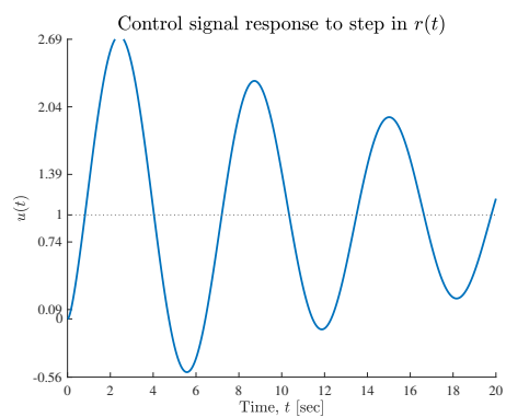
(ב) תגובת אות הבקרה עבור צמצום של אפסים לא מרוסנים
