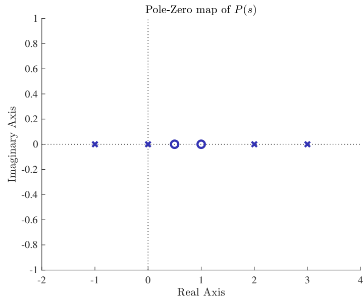
איור 14: מפת הקטבים של התהליך
