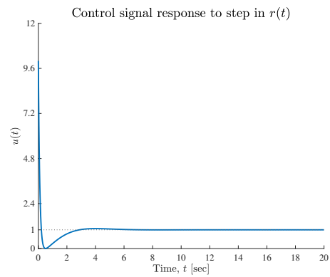
(ב) תגובת אות הבקרה עבור צמצום של קטבים לא מרוסנים
