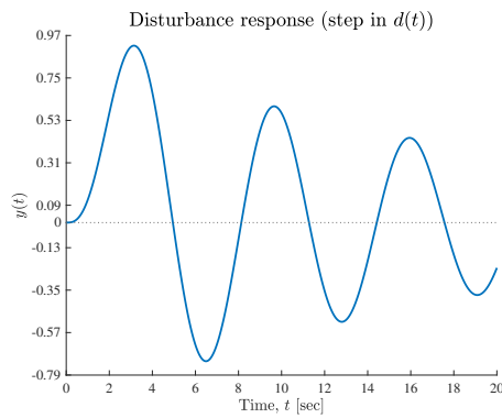
(א) תגובת ההפרעה עבור צמצום של קטבים לא מרוסנים
