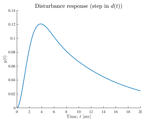
(א) תגובת ההפרעה עבור צמצום של קוטב איטי
