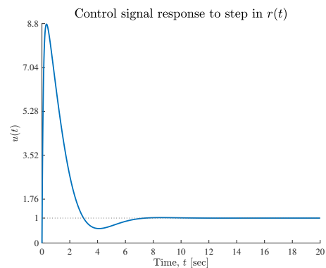
(ב) תגובת אות הבקרה עבור צמצום של קוטב איטי
