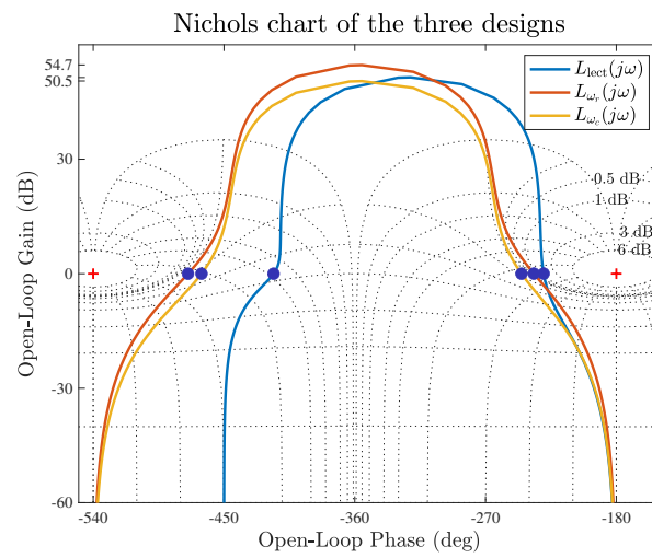
איור 5: עקומי ניקולס עבור שלושת החוגים
