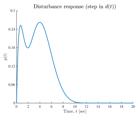
(א) תגובת ההפרעה עבור צמצום של אפסים לא מרוסנים
